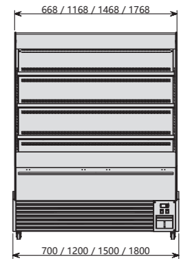
正视图 Front View
